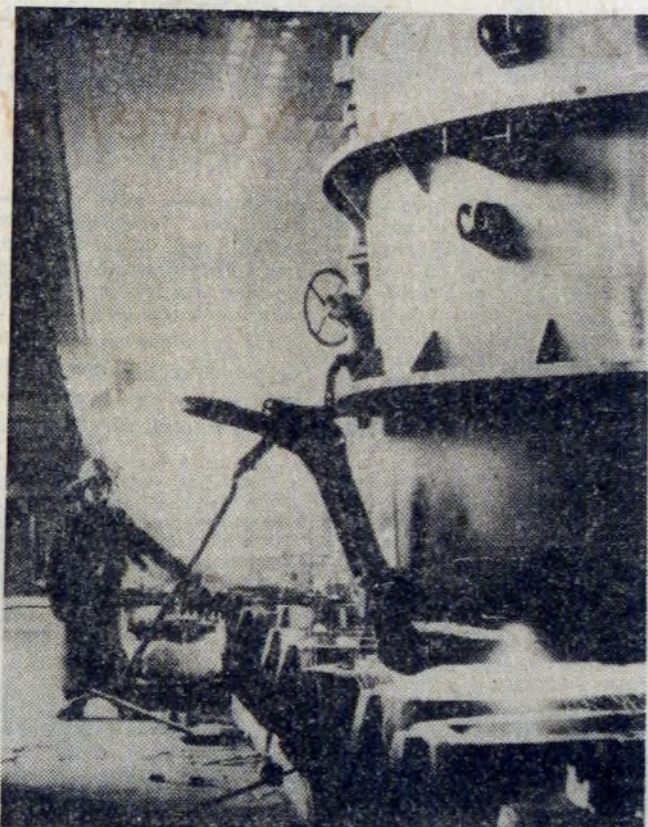
Jakże niepozornie wygląda człowiek przy tych wielkich urządzeniach Stalowni Konwertorowej. A przecież właśnie ludzie decydują o wynikach pracy hutniczego kolosa... FOT. M. GLADYSEK
