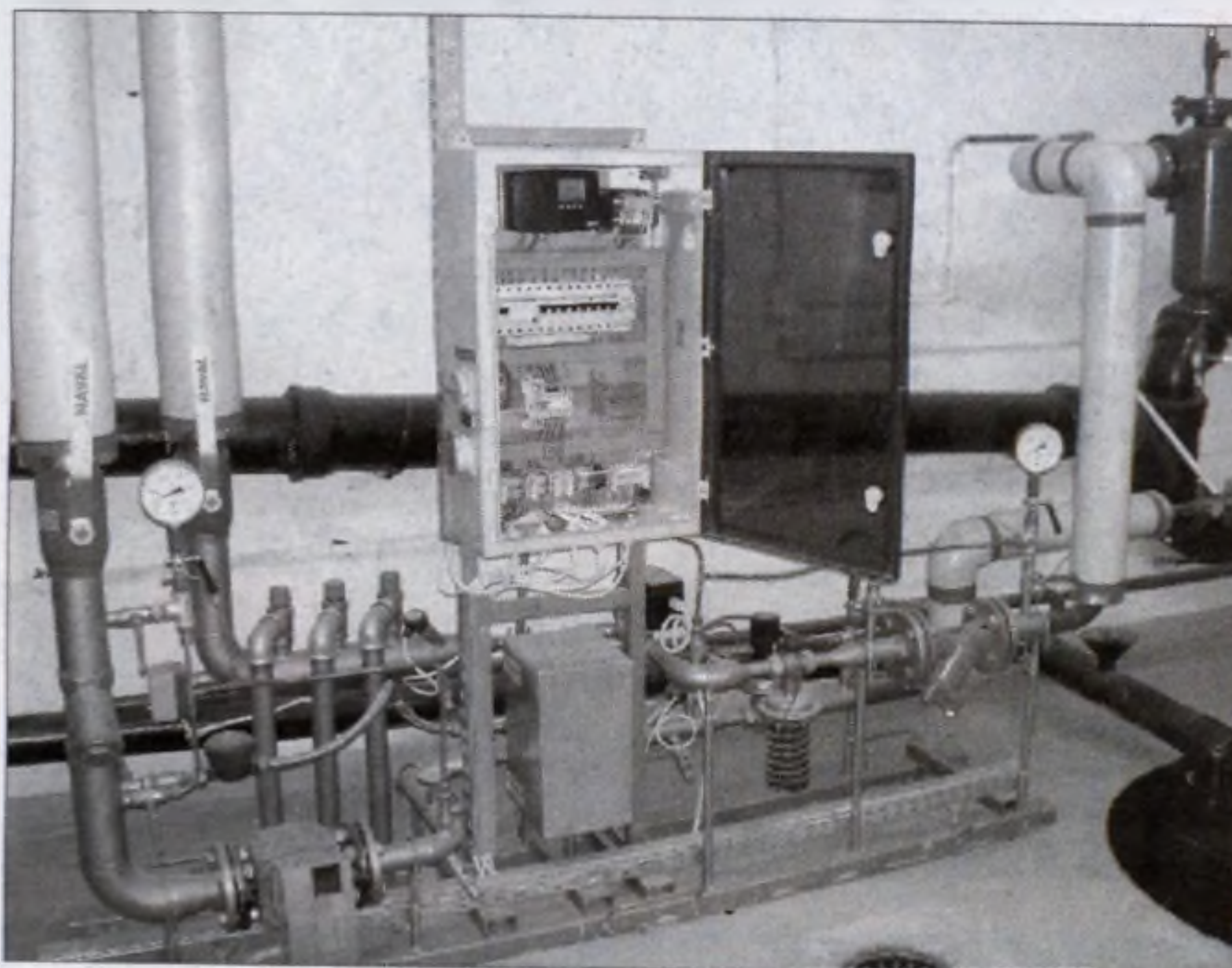
Nowoczesny węzeł zamontowany w budynku wielomieszkaniowym i sprzężony z automatyką pogodową gwarantuje oszczędne i efektywne ogrzewanie mieszkań.
